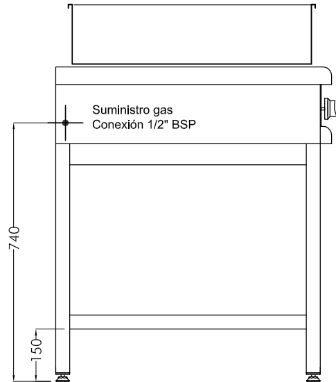
VISTA LATERAL ESC. 1:15
