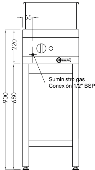
VISTA FRONTAL ESC. 1:15
