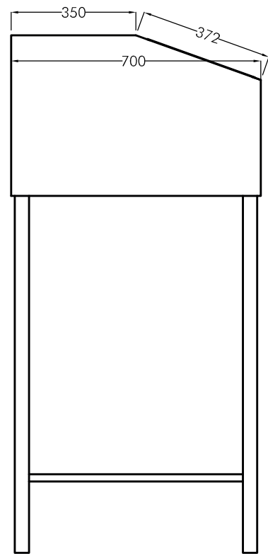
VISTA LATERAL
