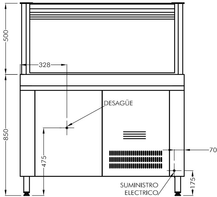
VISTA FRONTAL ESC. 1:20
